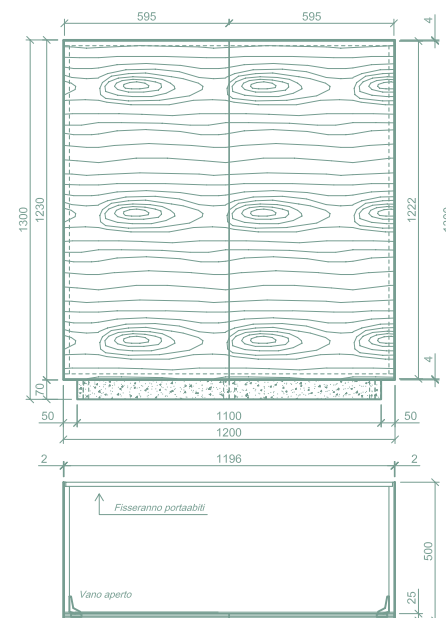
SEZ. ORIZZONTALE
